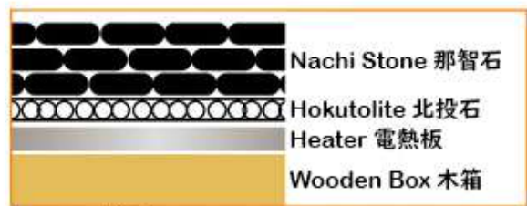
Section 剖面
